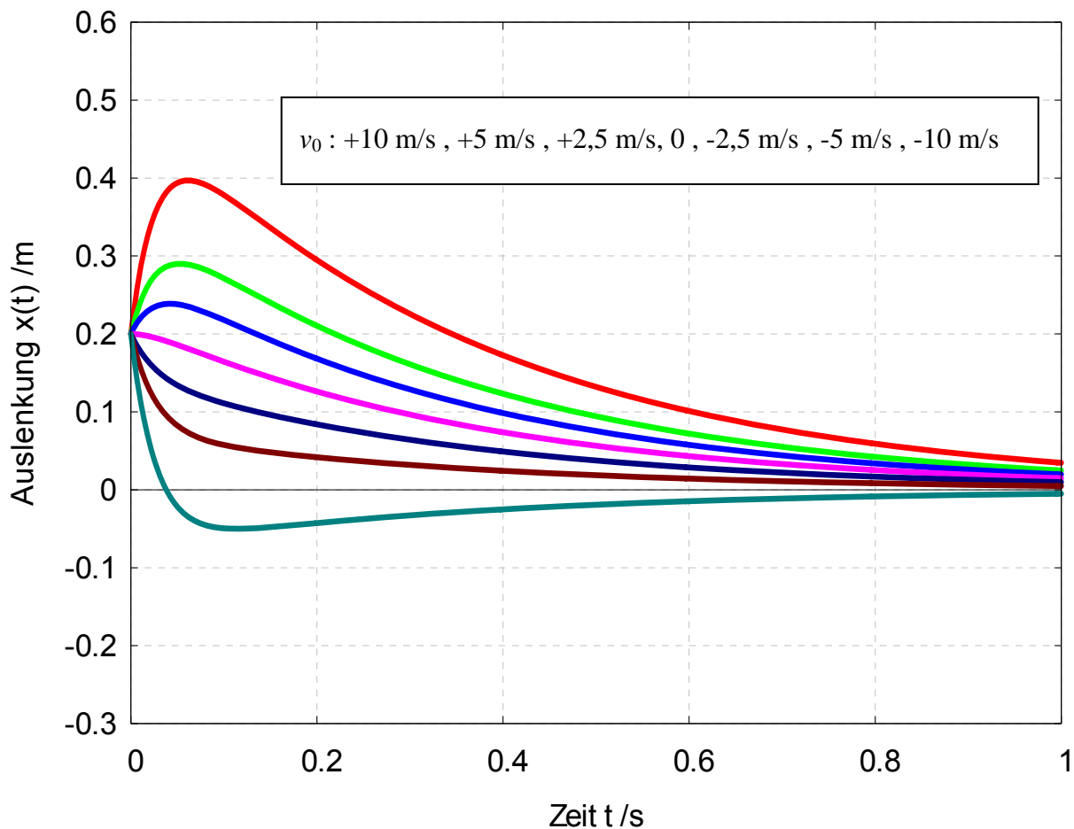
HO mit Daempfung, Kriechfall mit versch Anfangsgeschwindigkeiten
