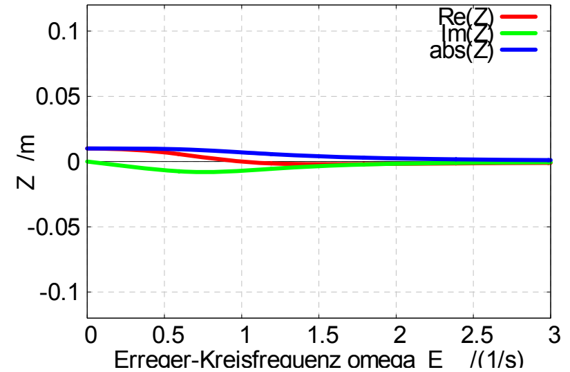
Erzwungene Schwingungen, Resonanz ; D = 0.707
